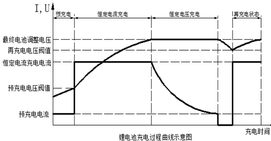
图 3.1.2 锂电池充电曲线图
