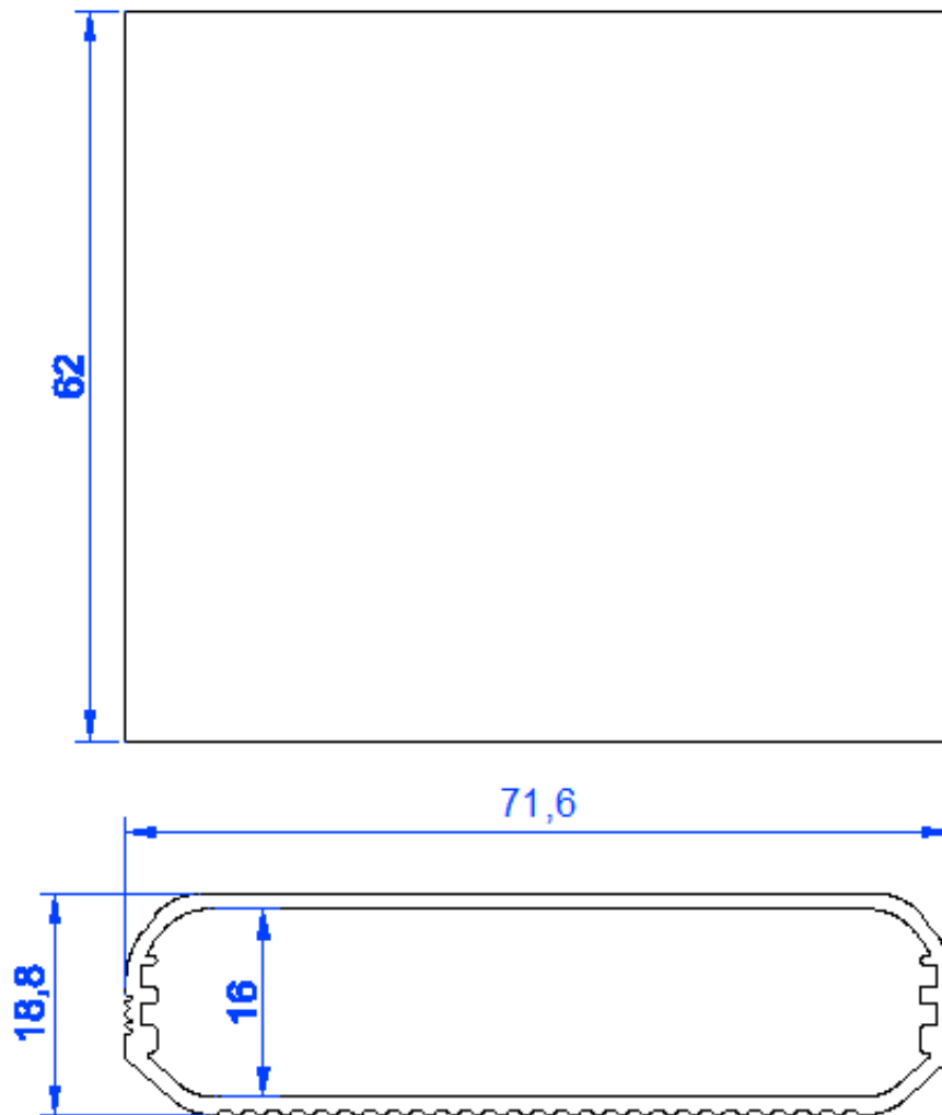
图 1.4 : 产品外观尺寸
