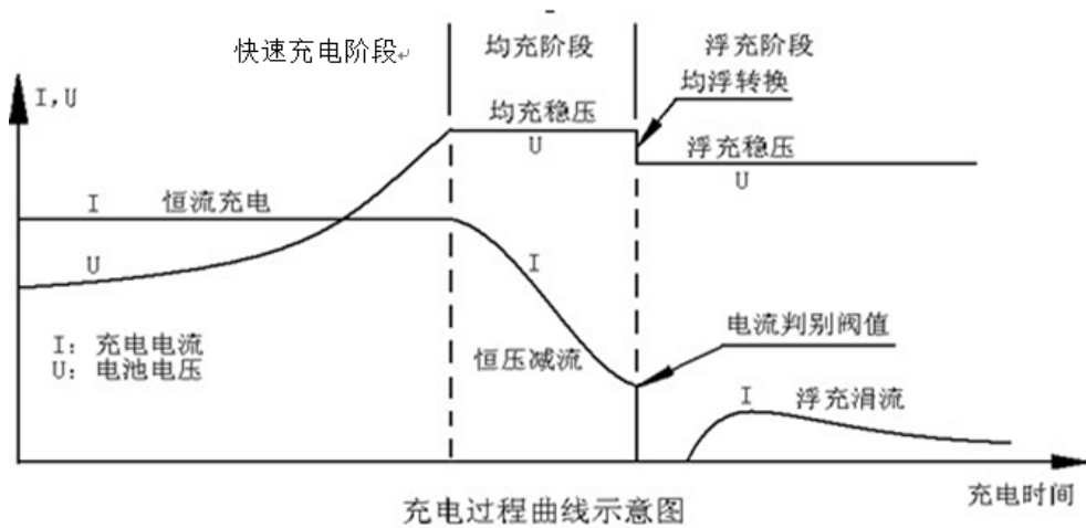
图 3.1.1 铅酸/胶体蓄电池充电曲线图
